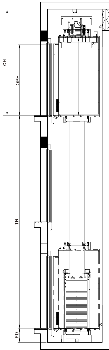
HOISTWAY ELEVATION
